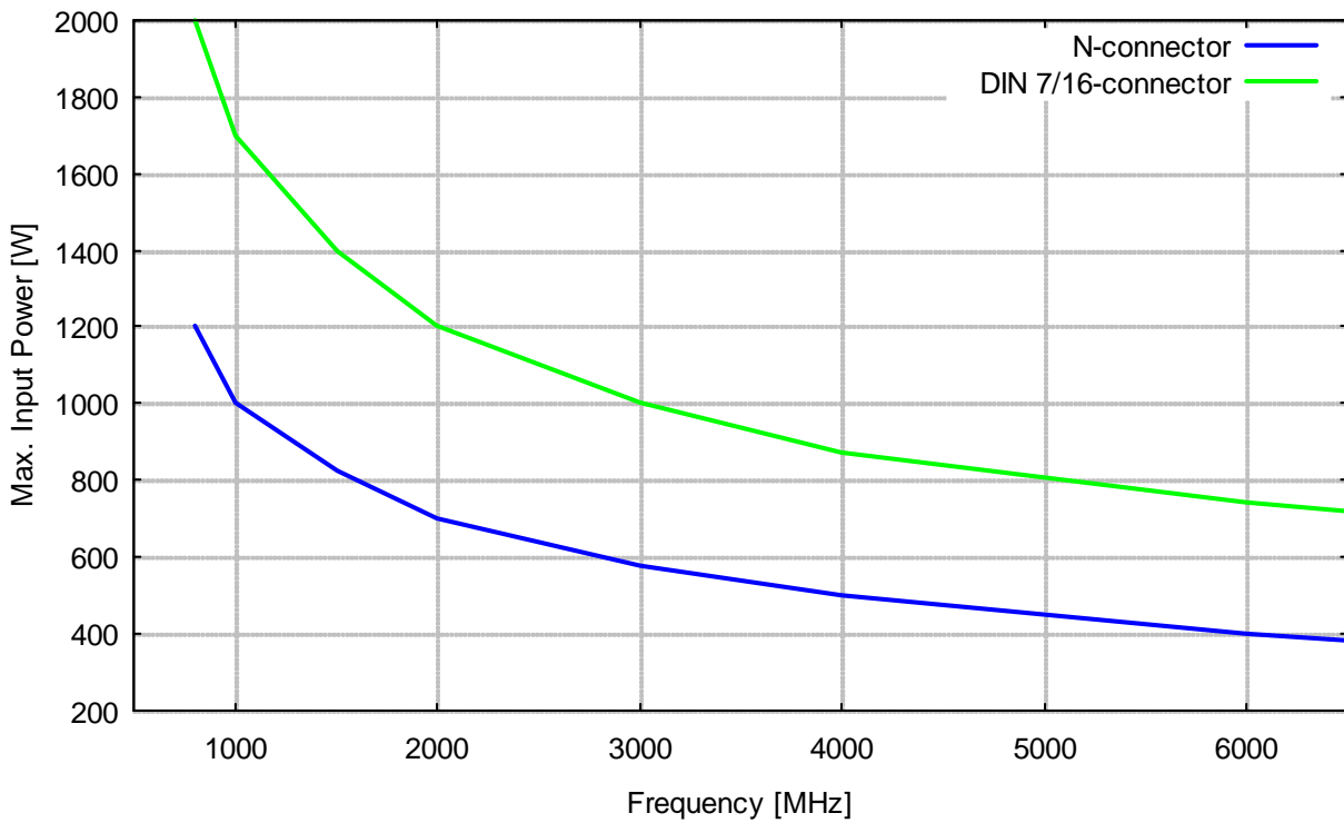
Maximale Eingangsleistung
