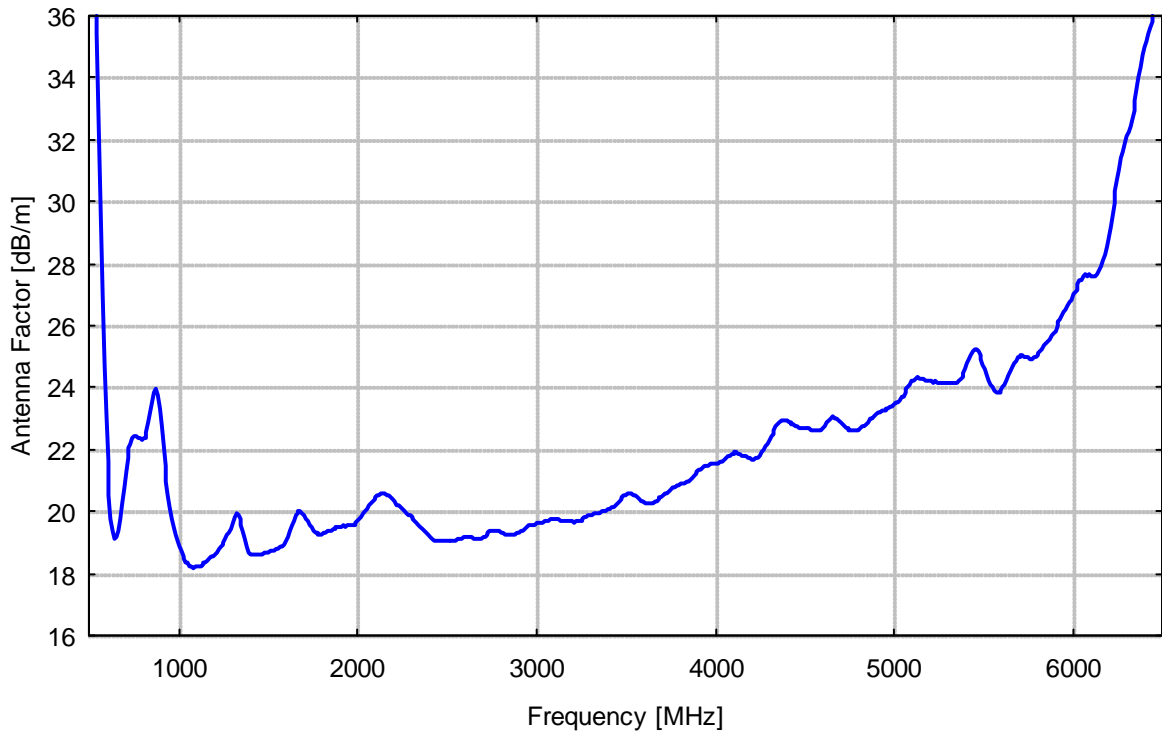
Antennen-Wandlungsmaß
